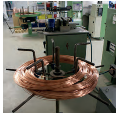
vollautomatisierte Ringproduktion fully automated ring production
