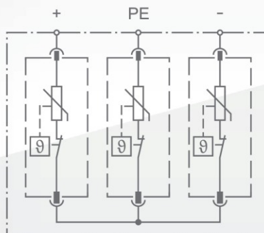
SCHEMA ZAPOJENÍ
