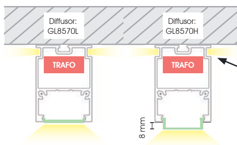
Aufbauversion /surface-mounted
