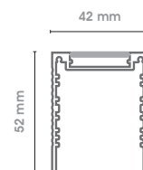
ALUPROFIL /aluminum profile
