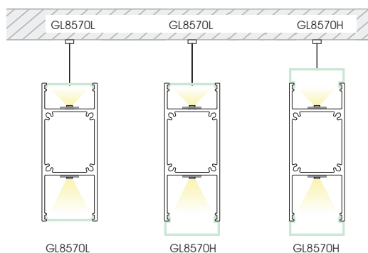
Pendelleuchte /pending lamp
