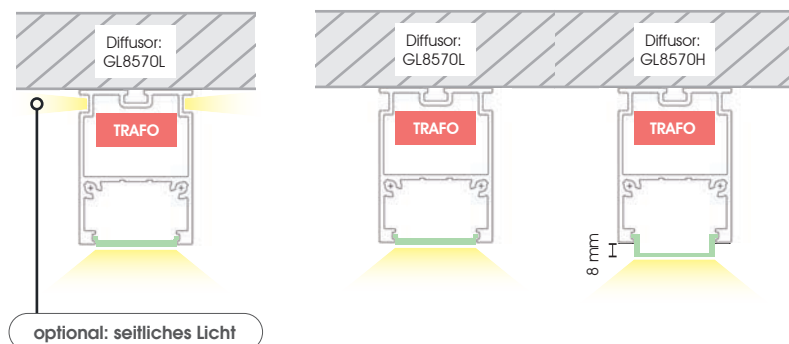
Aufbauversion / surface-mounted
